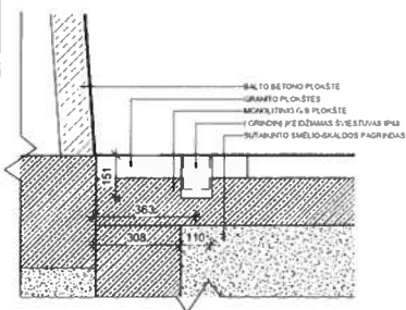
DETALĖ (D2) M1:20
